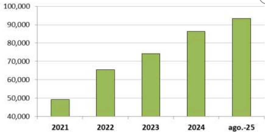
BPA
